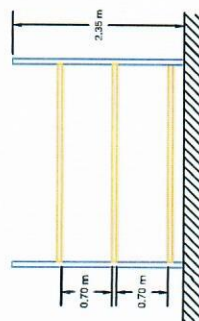
VISTA FRONTAL ESTANTERIA CARGAS MEDIAS 1500X600, 3 Niveles de Almacenaje, Capacidad de Carga 400 Kg por Nivel.
